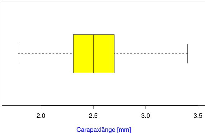
Boxplot, einfache Ausführung
