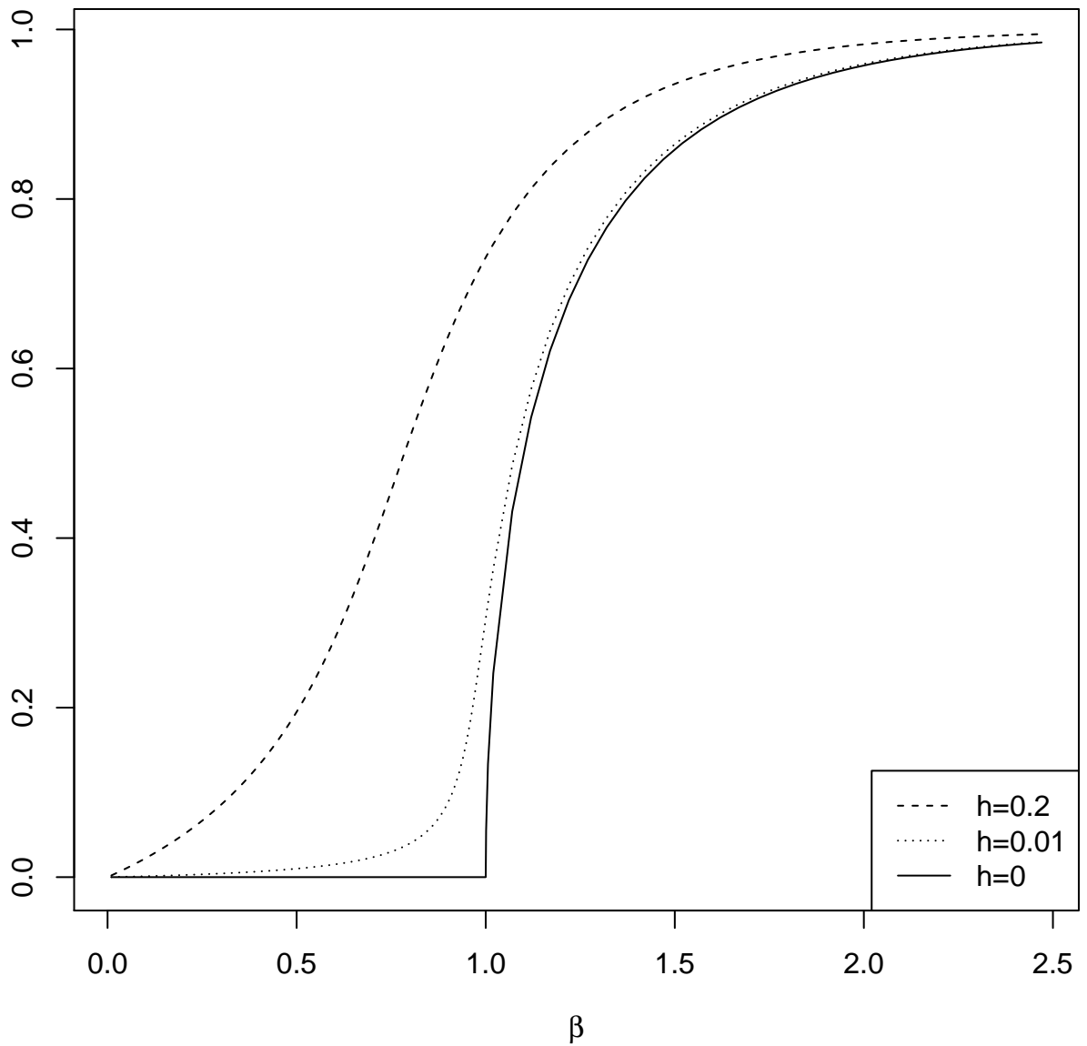
Mittlere Magnetisierung als Funktion von \beta
