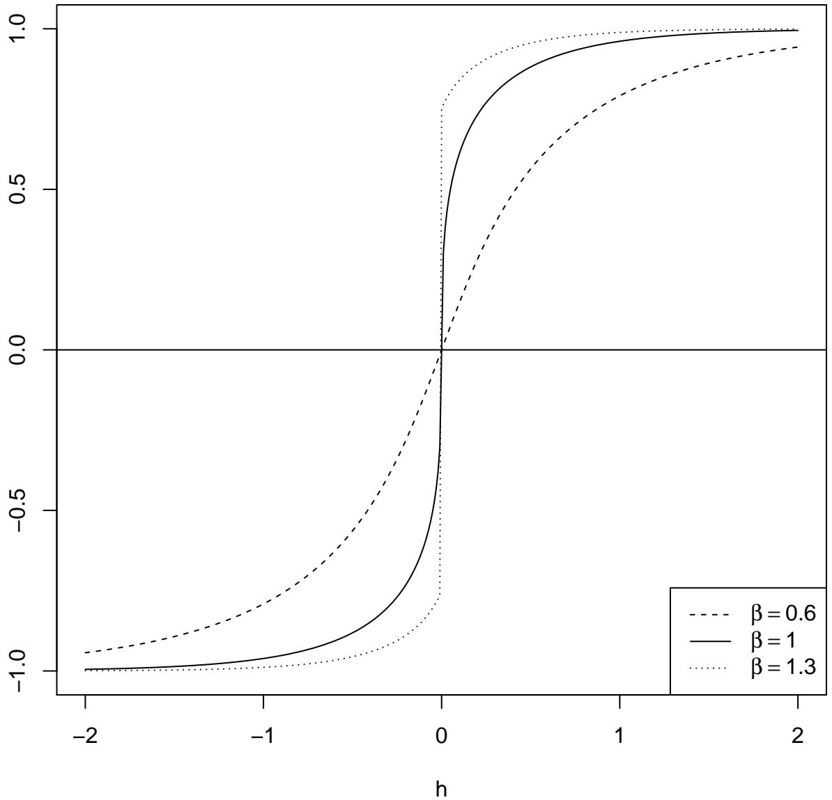
Mittlere Magnetisierung als Funktion von h
