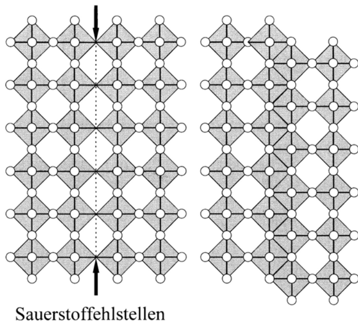
Perovskit-Struktur
