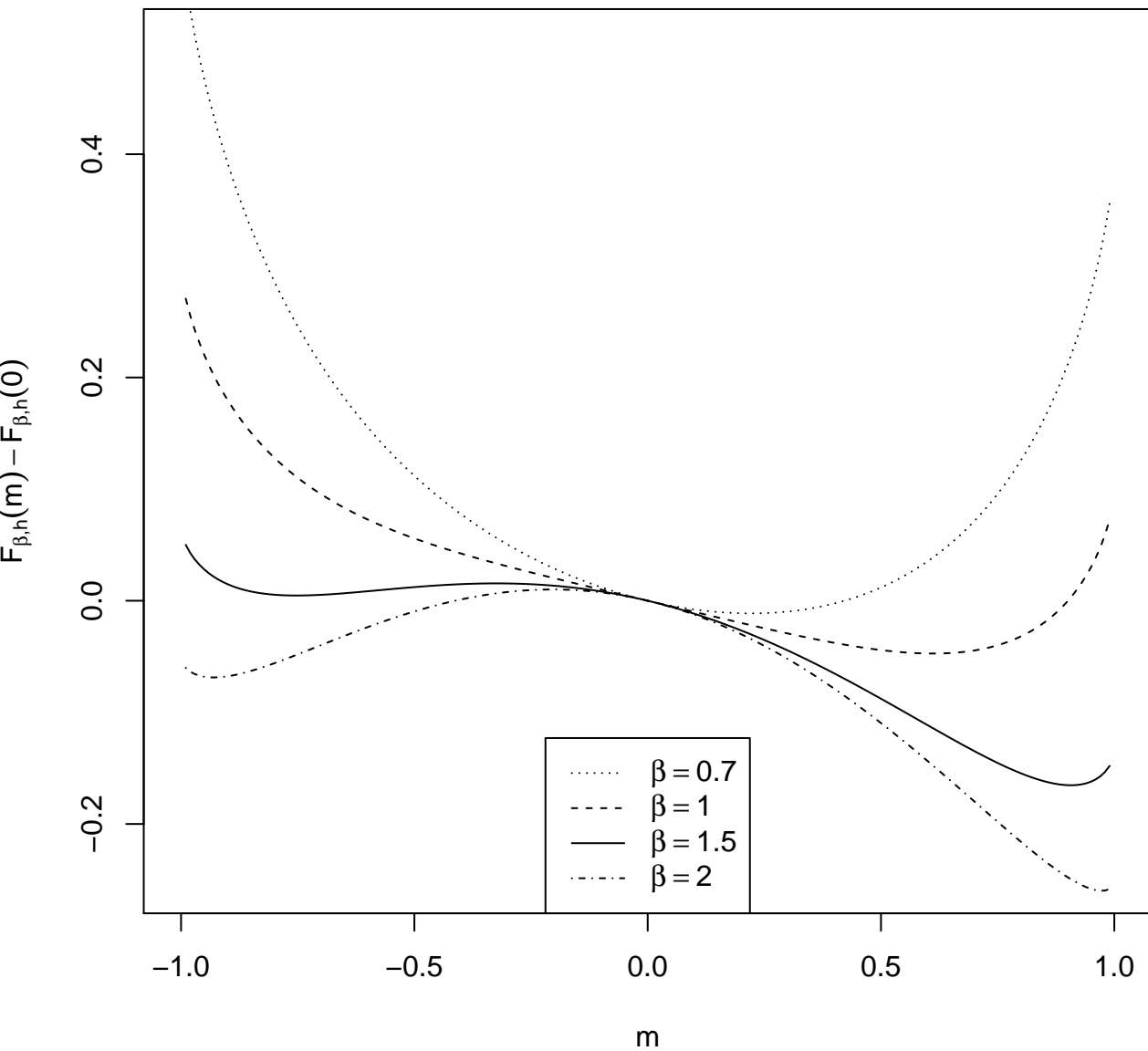
F_{\beta,h}(m) - F_{\beta,h}(0) als Funktion von m mit h = 0.1
