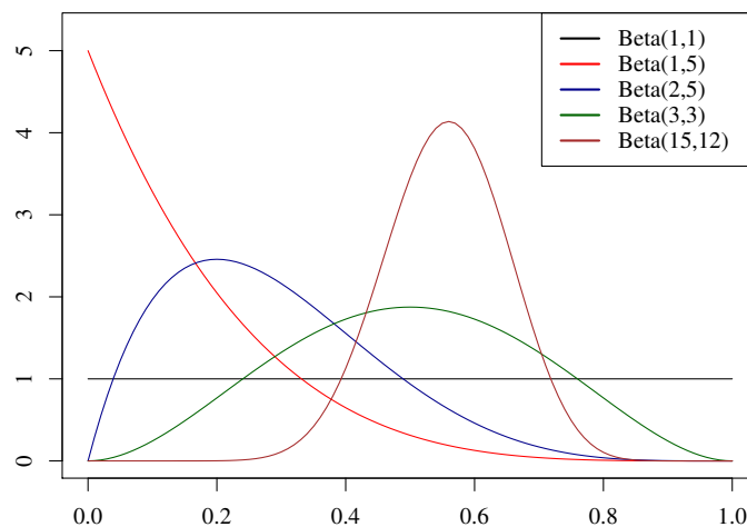
Einige Beta-Dichten:
