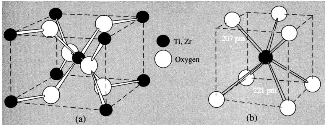
Rutil-Struktur
