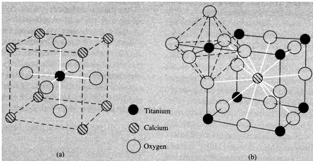
Perowskit-Struktur
