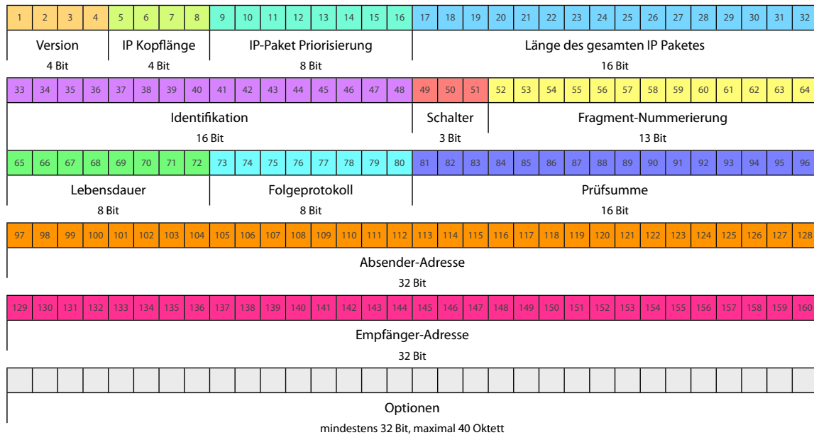
Abbildung 3.2: Aufbau des Kopfdatenbereichs eines IP-Paketes. Die einzelnen Zahlen in den Kästchen geben die Bitposition wider. Die Daten werden in aufsteigender Bit-Reihenfolge gesendet. Die Bitpositionen sind zu mehreren Bereichen zusammengefasst, welche unterschiedliche Bedeutungen und Funktionen besitzen.
