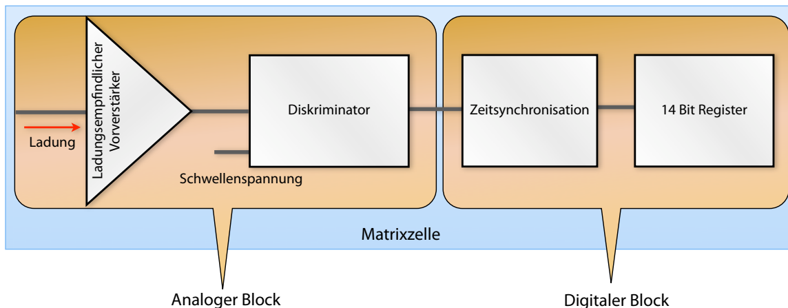
Abbildung 2.3: Schematische Darstellung der Arbeitsweise der Matrixzellen
