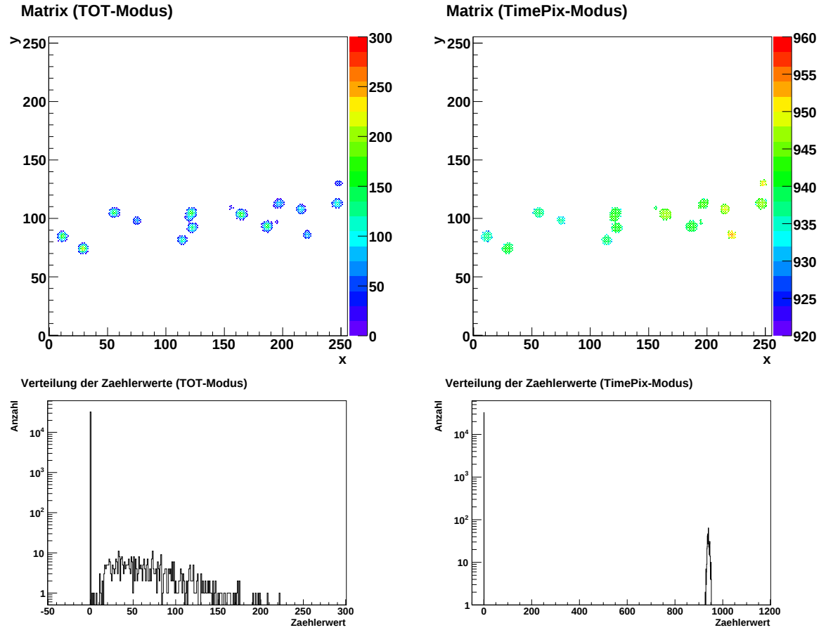
Abbildung 6.3: Spur eines kosmischen Teilchens, aufgenommen bei einer Schwelle ( \text{THL} ) von 348. Oben ist das Bild der Spur jeweils im TOT-Modus (links) bzw. Ankunftszeit-Modus (rechts) dargestellt. Unten werden die dazugehörigen Verteilungen der Zählstände gezeigt. Die Entfernung der Spur zur Ausleseebene betrug ungefähr s_{\text{Drift}} \approx 12,45 cm.
