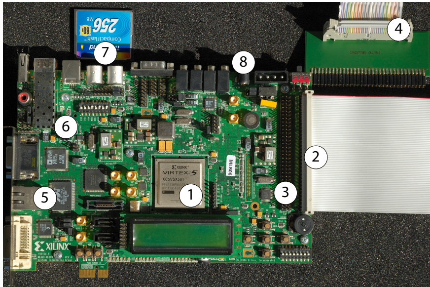
Abbildung 4.4: Foto der Xilinx Entwicklungsplatine mit FPGA. Mit Ziffern versehen sind: (1) der FPGA, (2) die Stiftleiste für CMOS-Signale, (3) die Stiftleiste für differentielle Signale, (4) das Flachkabel mit gedrehten Adernpaaren angeschlossen an den 63-auf-34-Adapter, (5) die PHY für den Ethernet-Anschluss, (6) der JTAG-Konfigurationsanschluss, (7) die CompactFlash Speicherkarte (der Anschluss befindet sich auf der Rückseite der Platine) und (8) der 5 V Versorgungsspannungsanschluss.
