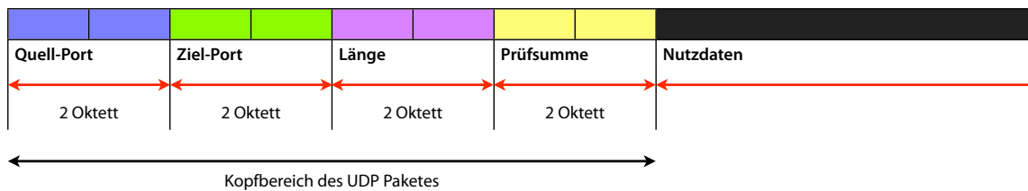
Abbildung 3.3: Aufbau des Kopfdatenbereichs eines UDP-Paketes, bestehend aus dem Quell-Post und dem Ziel-Post, der Paketlänge und der optionalen Prüfsumme. Die einzelnen Daten werden in aufsteigender Oktett-Reihenfolge verschickt.
