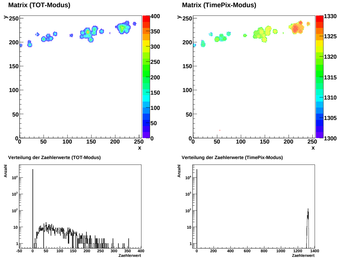
Abbildung 6.6: Spur eines kosmischen Teilchens, aufgenommen bei einer Schwelle ( \text{THL} ) von 348. Oben ist das Bild der Spur jeweils im TOT-Modus (links) bzw. Ankunftszeit-Modus (rechts) dargestellt. Unten werden die dazugehörigen Verteilungen der Zählstände gezeigt. Die Entfernung der Spur zur Ausleseebene betrug ungefähr s_{\text{Drift}} \approx 4,40 cm.
