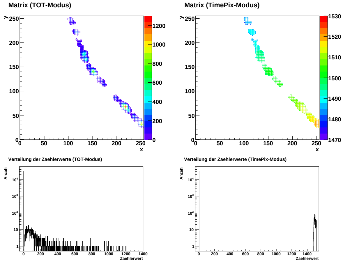
Abbildung 6.10: Spur eines kosmischen Teilchens, aufgenommen bei einer Schwelle ( \text{THL} ) von 348. Oben ist das Bild der Spur jeweils im TOT-Modus (links) bzw. Ankunftszeit-Modus (rechts) dargestellt. Unten werden die dazugehörigen Verteilungen der Zählstände gezeigt. Die Entfernung der Spur zur Ausleseebene betrug ungefähr s_{\text{Drift}} \approx 0,21 cm.
