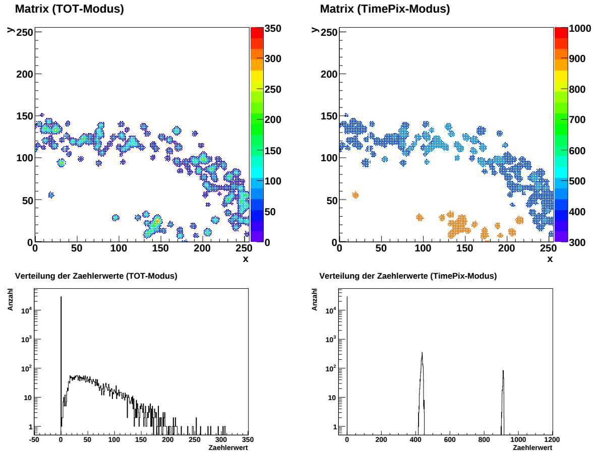
Abbildung 6.11: Spur eines kosmischen Teilchens, aufgenommen bei einer Schwelle ( \text{THL} ) von 348. Oben ist das Bild der Spur jeweils im TOT-Modus (links) bzw. Ankunftszeit-Modus (rechts) dargestellt. Unten werden die dazugehörigen Verteilungen der Zählstände gezeigt. Die Entfernung der Spur zur Ausleseebene betrug ungefähr s_{\text{Drift}} \approx 13,52 cm. Innerhalb der Blendenöffnungszeit wurde ein Teil einer zweiten Spur aufgezeichnet.
