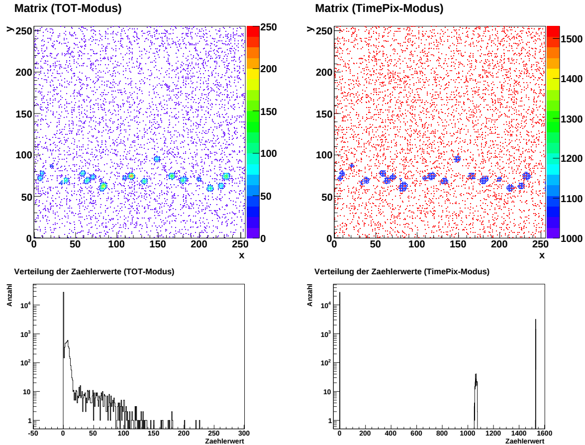
Abbildung 6.8: Spur eines kosmischen Teilchens, aufgenommen bei einer Schwelle ( THL ) von 330. Oben ist das Bild der Spur jeweils im TOT-Modus (links) bzw. Ankunftszeit-Modus (rechts) dargestellt. Unten werden die dazugehörigen Verteilungen der Zählstände gezeigt. Die Entfernung der Spur zur Ausleseebene betrug ungefähr s_{\text{Drift}} \approx 9,23 cm. Bei dieser Aufnahme erkennt man das deutliche Rauschen, welches sich in den zwei Spitzen beider Verteilungen widerspiegelt.
