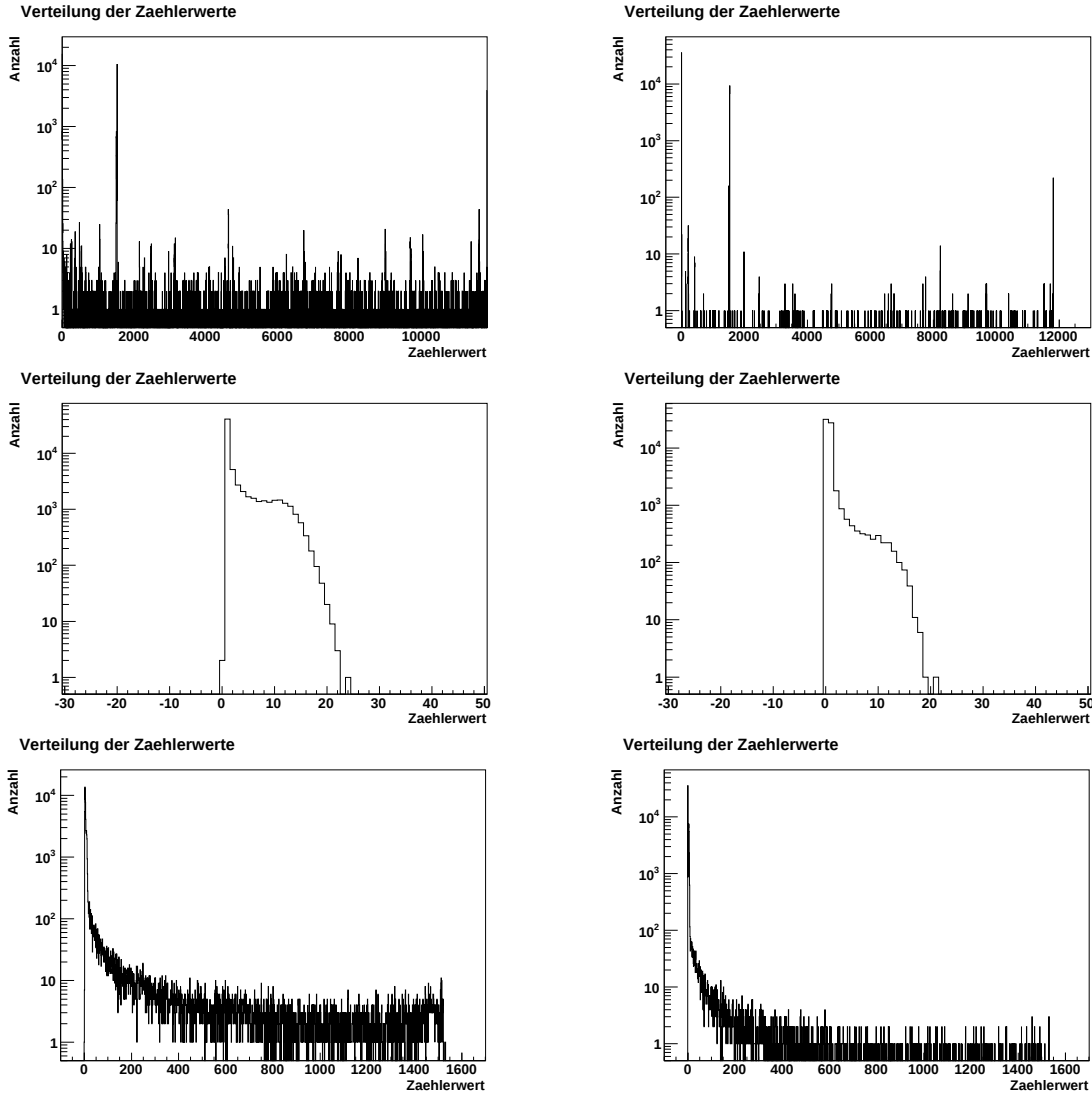
Abbildung 5.9: Darstellung der Zählstände nach Aufnahme vom Rauschen im Ankunftszeit-, Ereigniszähl- und TOT-Modus bei den Schwellen ( T_{HL} ) von 290 und 330. Links sind alle Bilder bei der Schwelle von 290 dargestellt, rechts bei der Schwelle von 330. Die Bilder oben sind im Ankunftszeit-Modus, die Bilder in der Mitte im Ereigniszähl-Modus und die unteren Bilder im TOT-Modus. In Abbildung 5.10 werden die dazugehörigen Matrixbilder gezeigt. Alle Bilder wurden bei einer Betriebsfrequenz von \nu_{Takt} = 40 MHz und einer Blendenöffnungszeit von t_1 = 38,25 \mu s aufgenommen.
